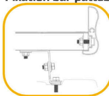
Fixation sur pattes
