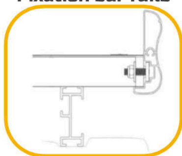
Fixation sur rails
