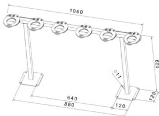
Fixation range trottinettes sur pied
