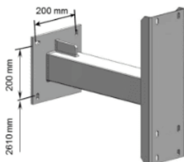
Implantation à 2,60m
