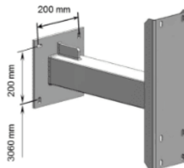
Implantation à 3,05m
